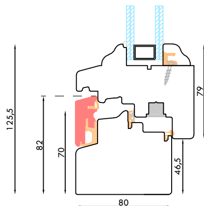
NODO INFERIORE FINESTRA CON GOCCIOLATOIO A BECCO
