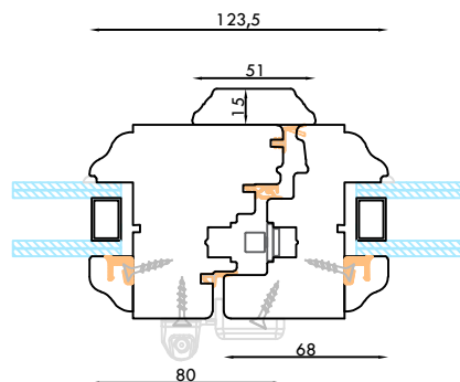
NODO CENTRALE TERZA ANTA
