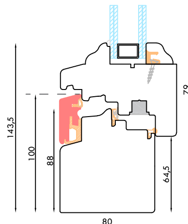
NODO INFERIORE FINESTRA CON GOCCIOLATOIO A BECCO E TRAVERSO INFERIORE MAGGIORATO
