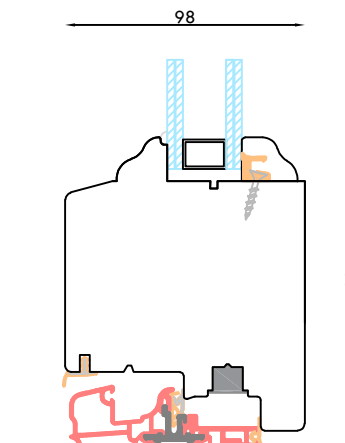
NODO INFERIORE FINESTRA CON GOCCIOLATOIO A BECCO E TRAVERSO INFERIORE MAGGIORATO
