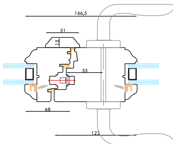
NODO CENTRALE CON MANIGLIA PASSANTE, LISTA CENTRALE LISCIA E MONTANTE DELLA SERRATURA MAGGIORATO 118 x 80
