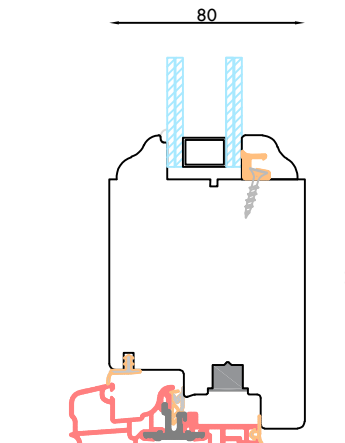
NODO INFERIORE PORTA FINESTRA CON SOGLIA STD E ZOCCOLO UNICO DA 120 mm
