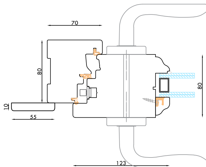
NODO LATERALE CON MANIGLIA PASSANTE, MONTANTE ANTA MAGGIORATO
