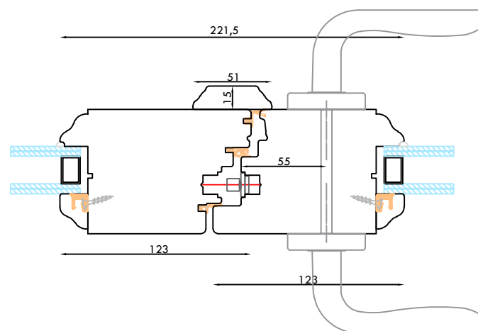
NODO CENTRALE CON MANIGLIA PASSANTE, LISTA CENTRALE LISCIA ED ENTRAMBE I MONTANTI MAGGIORATI 118x80
