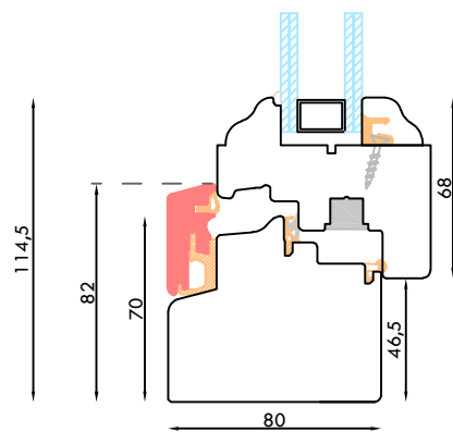
NODO INFERIORE FINESTRA CON GOCCIOLATOIO
