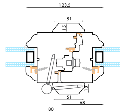
NODO CENTRALE TERZA ANTA CON LISTA ENTRATA O SAGOMATA PER CERNIRE ANUBA
