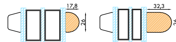
DIMENSIONI MINIME
