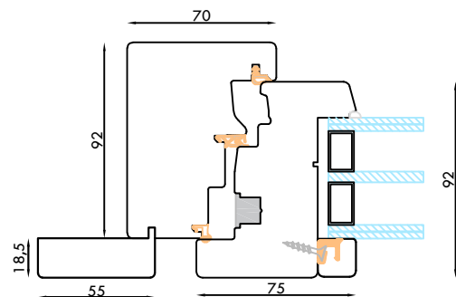
TELAIO LINEO CON COPRIFILO COMPLANARE ALL'ANTA
