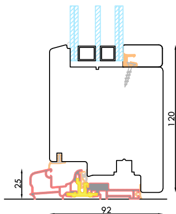
NODO INFERIORE PORTA FINESTRA CON SOGLIA STD E ZOCCOLO UNICO DA 120 mm
