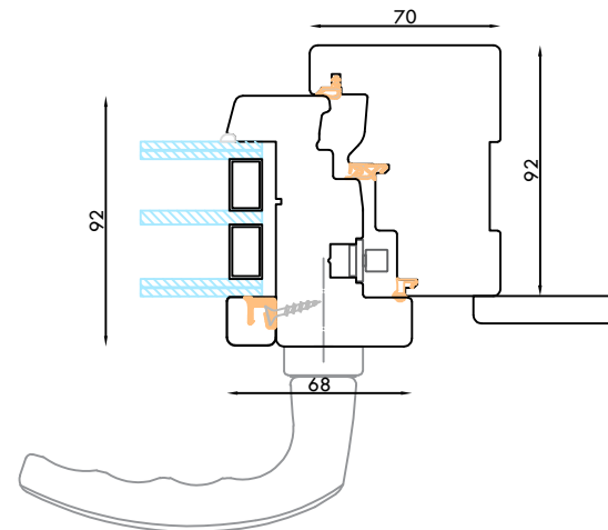
NODO CENTRALE RISTRETTO
