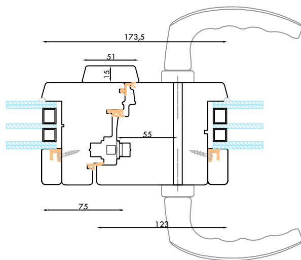
NODO CENTRALE CON MANIGLIA PASSANTE (YALE) ASIMMETRICO MONTANTI MAGGIORATI
