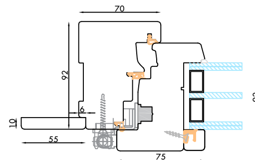
TELAIO FLAT CON ALLOGGIAMENTO DA 10 x 6 mm PER COPRIFILO COMPLANARE AL TELAIO
