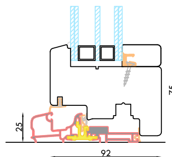
NODO INFERIORE PORTA FINESTRA CON SOGLIA STD E ZOCCOLO UNICO DA 75 mm
