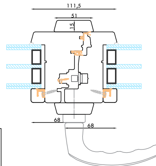
NODO CENTRALE RISTRETTO
