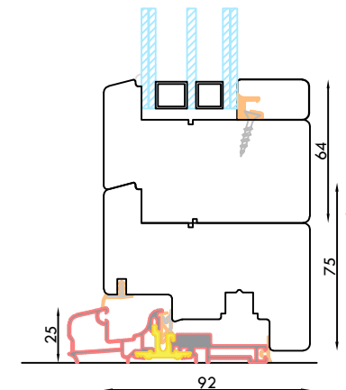
NODO INFERIORE PORTA FINESTRA CON SOGLIA STD E DOPPIO ZOCCOLO DA 121 mm
