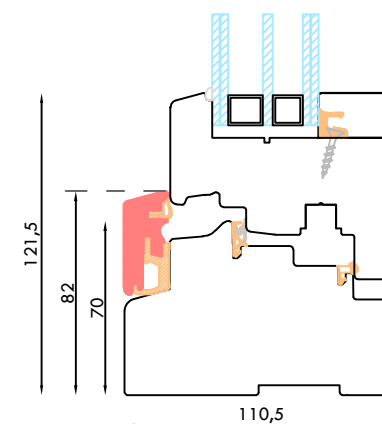
NODO INFERIORE FINESTRA CON GOCCIOLATOIO E TELAIO PLANEO
