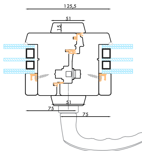
NODO CENTRALE SIMMETRICO CON LISTA INTERNA
