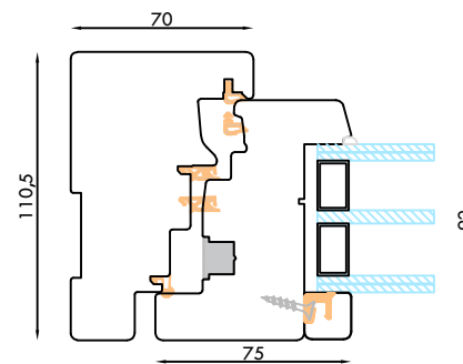
TELAIO PLANO, COMPLANARE ALL'ANTA
