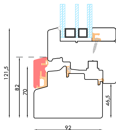
NODO INFERIORE FINESTRA CON GOCCIOLATOIO
