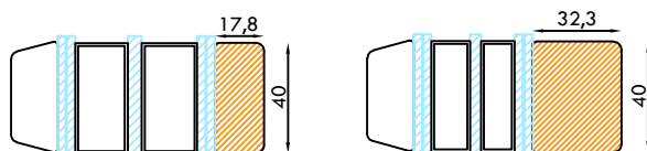
DIMENSIONI MASSIME
