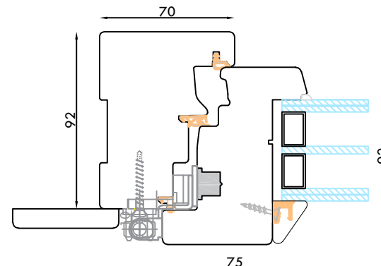
PROFILO INFINITO
