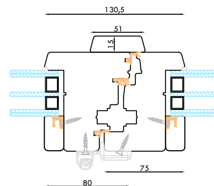
NODO CENTRALE TERZA ANTA
