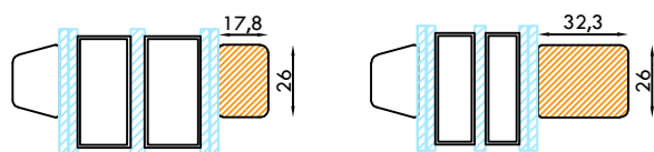
DIMENSIONI MINIME
