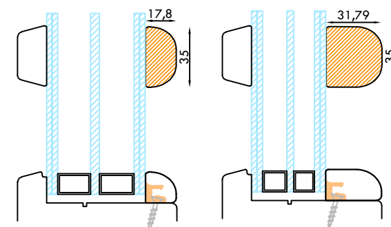
PROFILO RONDO'
