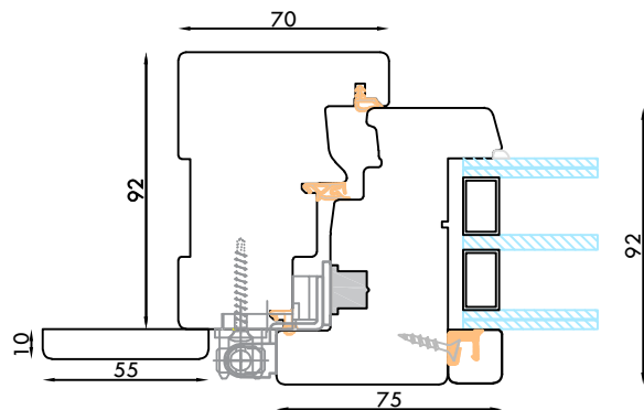
NODO LATERALE CON CERNIERA
