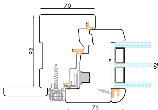
PROFILO RONDO'
