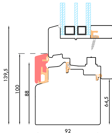
NODO INFERIORE FINESTRA CON GOCCIOLATOIO
