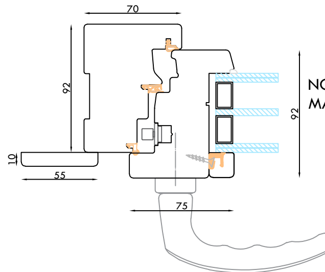
Tipologie profili
