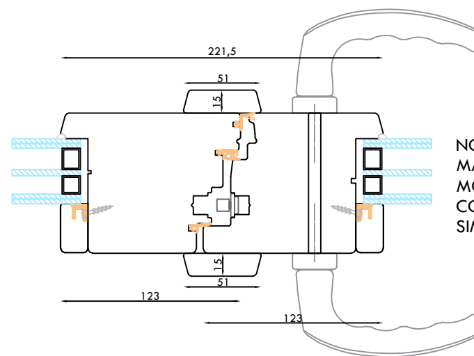
NODO CENTRALE CON MANIGLIA PASSANTE (YALE) ASIMMETRICO MONTANTI MAGGIORATI
