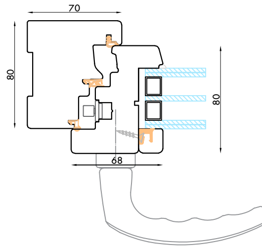
SEZIONE ANTA MINIMAL 68 x 80 mm
