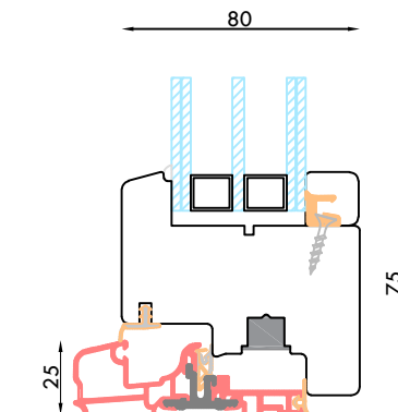
NODO INFERIORE PORTA FINESTRA CON SOGLIA STD CON ZOCCOLO UNICO DA 75 mm
