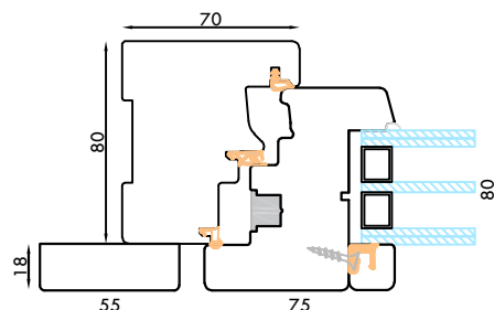
TELAIO LINEO, CON COPRIFILO COMPLANARE ALL'ANTA
