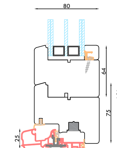
NODO INFERIORE PORTA FINESTRA CON SOGLIA STD CON DOPPIO ZOCCOLO DA 121 mm
