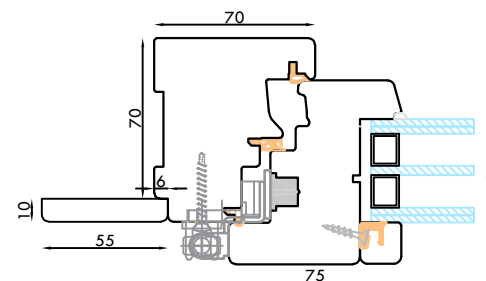
TELAIO FLAT, CON ALLOGGIO DA 10 x 6 mm PER COPRIFILO COMPLANARE AL TELAIO
