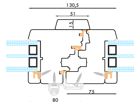
NODO CENTRALE TERZA ANTA
