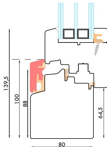
NODO INFERIORE FINESTRA CON GOCCIOLATOIO
