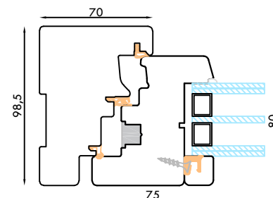
TELAIO PLANE, COMPLANARE ALL'ANTA
