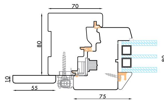
PROFILO INFINITO SPESSORE VETRO MASSIMO 40,5 mm
