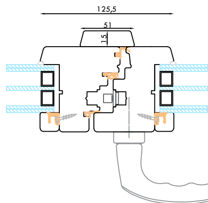
NODO CENTRALE ASIMMETRICO INTERNO E ESTERNO SIMMETRICO
