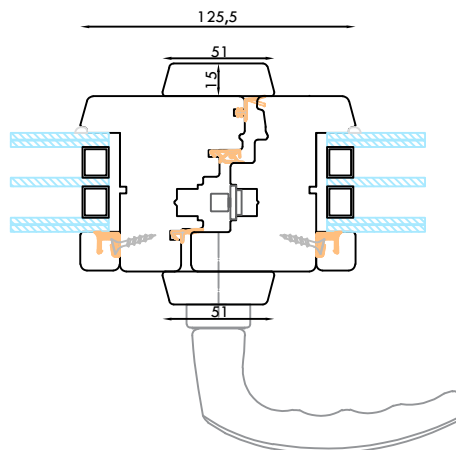
NODO CENTRALE SIMMETRICO SIA INTERNO CHE ESTERNO CON LISTA INTERNA
