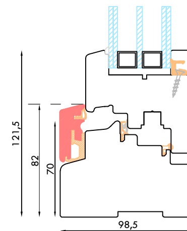
NODO INFERIORE FINESTRA CON GOCCIOLATOIO E TRAVERSO INFERIORE MAGGIORATO
