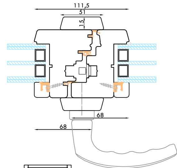
NODO CENTRALE RISTRETTO
