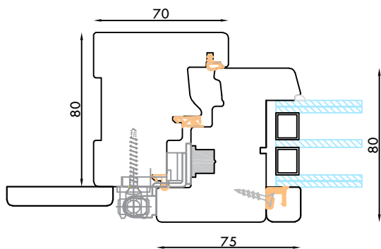
NODO LATERALE CON CERNIERA
