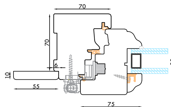
TELAIO FLAT, CON ALLOGGIO D A 10x6 PER COPRIFILO COMPLANARE AL TELAIIO
