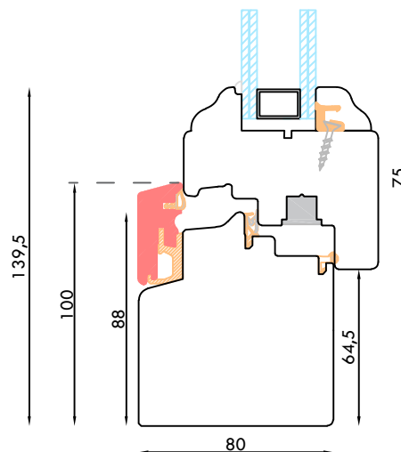
NODO INFERIORE FINESTRA CON GOCCIOLATOIO E TRAVERSO INFERIORE MAGGIORATO
