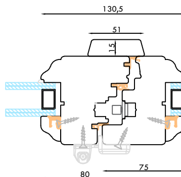
NODO CENTRALE SIMMETRICO CON LISTA CENTRALE ENTRATA O LISCIA
