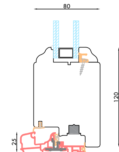
NODO INFERIORE PORTA FINESTRA CON SOGLIA STD E ZOCCHO UNICO DA 120 mm
