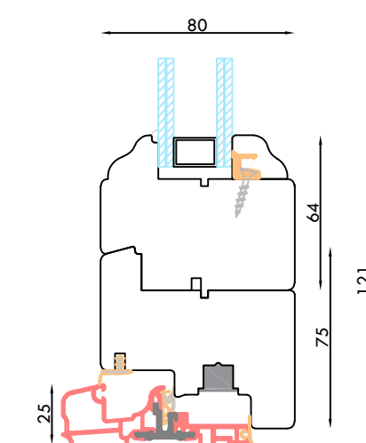
NODO INFERIORE PORTA FINESTRA CON SOGLIA STD E DOPPIO ZOCCHO DA 121 mm
