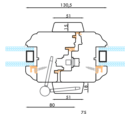
NODO CENTRALE TERZA ANTA CON LISTA ENTRATA O LISCIA PER CERNIRE ANUBA
