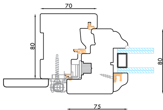
NODO LATERALE CON CERNIERA
