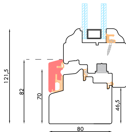
NODO INFERIORE FINESTRA CON GOCCIOLATOIO
