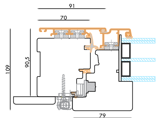
PROFILO ET-340
