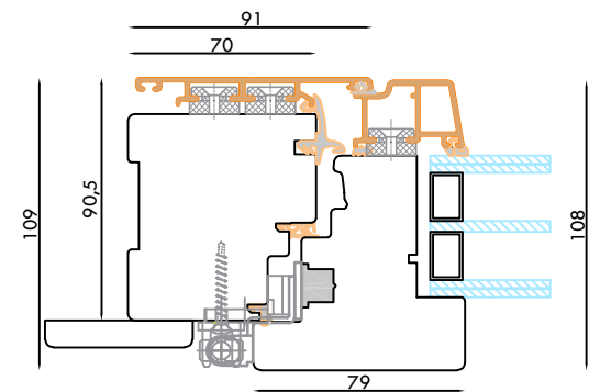
PROFILO ET-310
