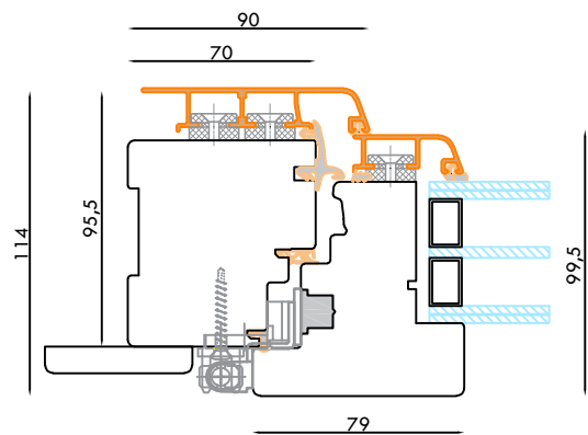
PROFILO R5
