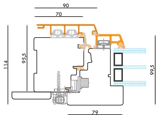
PROFILO R2
