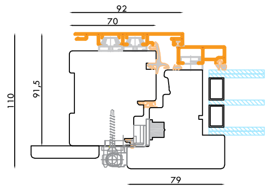
PROFILO 90
