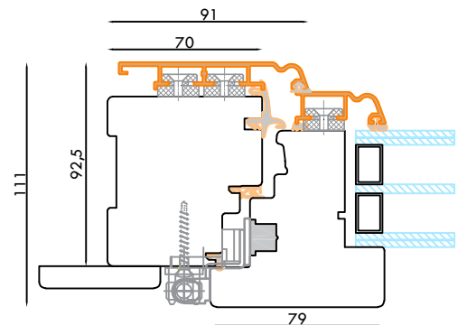
PROFILO ET-142
